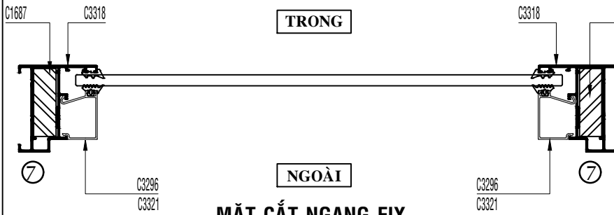
MẶT CẮT NGANG FIX
