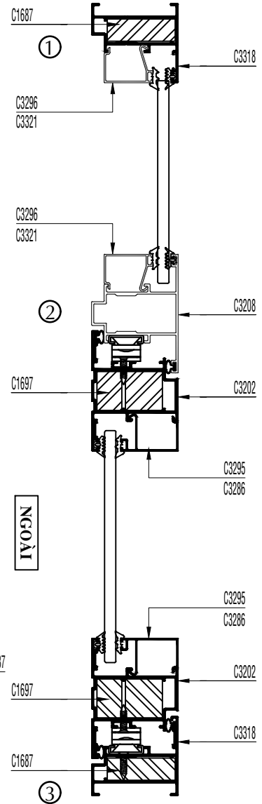
MẶT CẮT ĐỨNG
