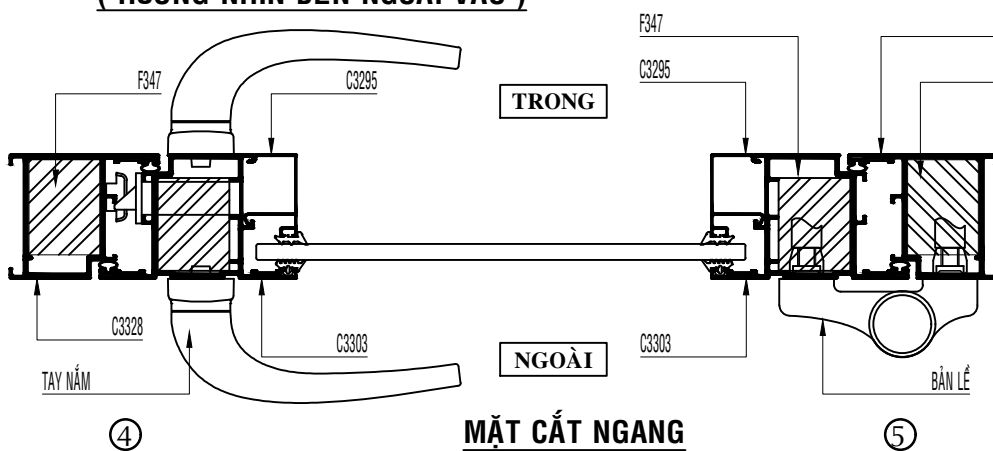
CỬA ĐI 1 CÁNH MỞ NGOÀI ( HƯỚNG NHÌN BÊN NGOÀI VÀO )
